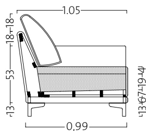
Vista corte lateral
