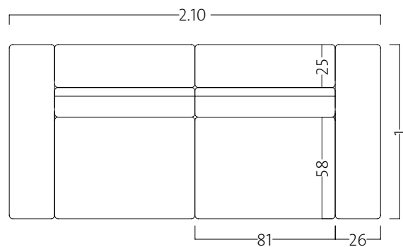
Vista superior
