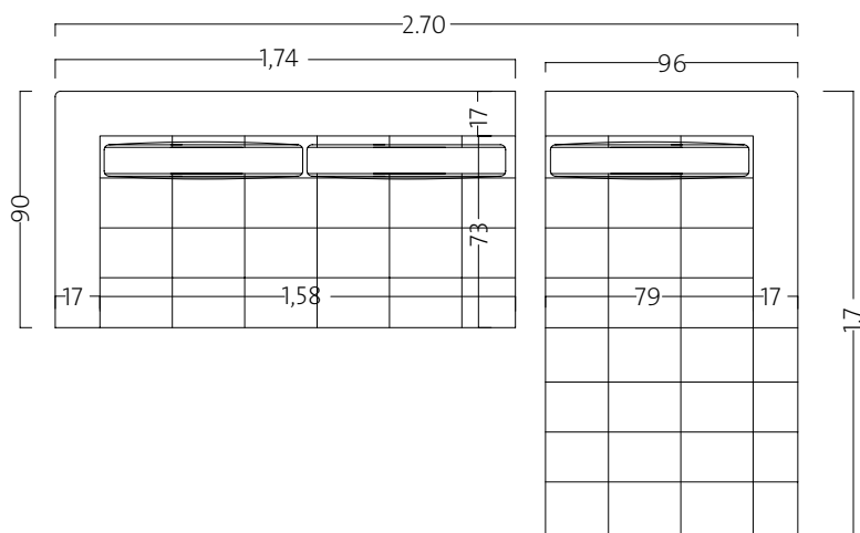
Vista superior
